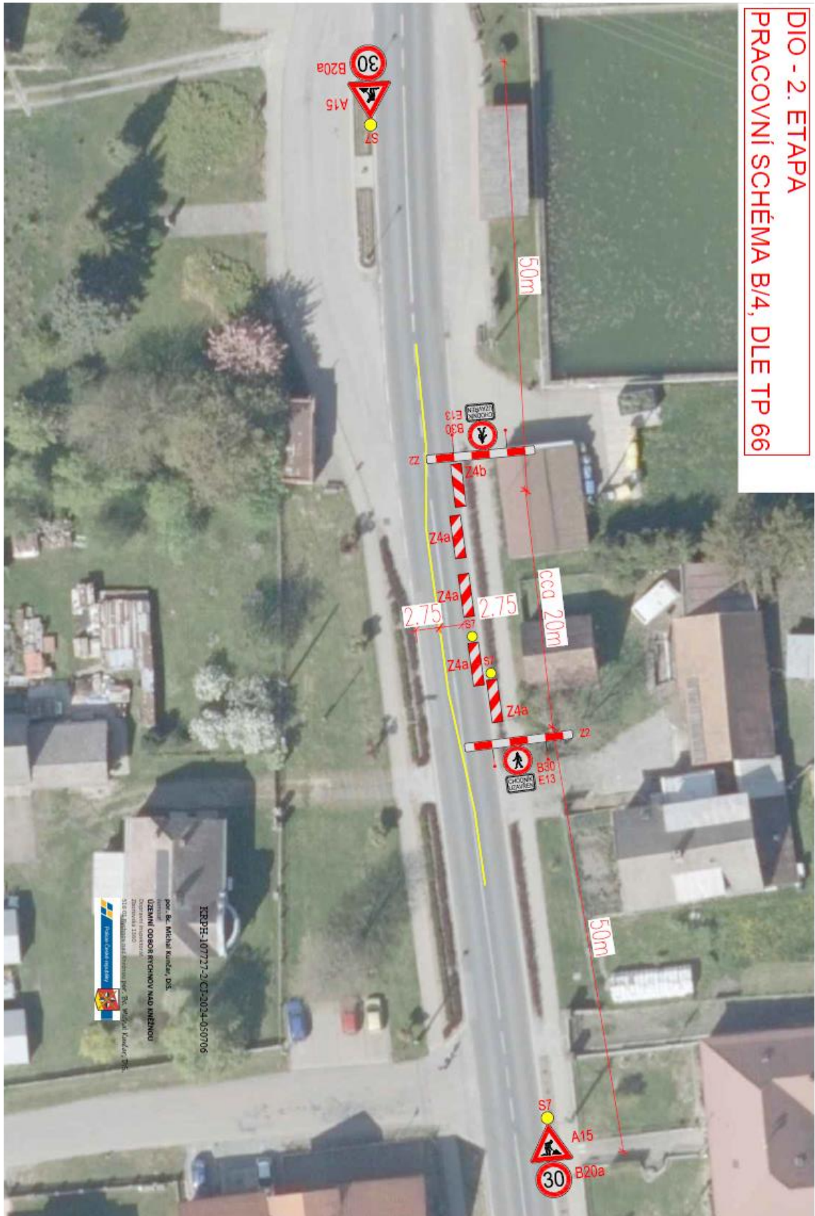
Situační schéma s vyznačeným umístěním přechodného dopravního značení
